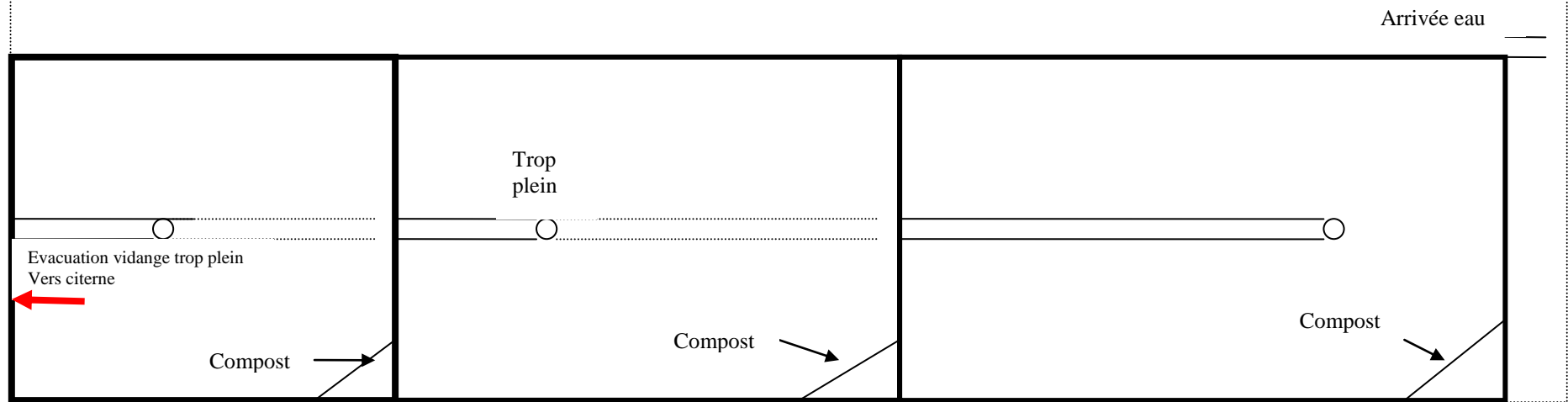
Document 12. Plan des bassins. Pisciculture Ecole Dumarsais Estimé. Verrettes Centre Bourg
